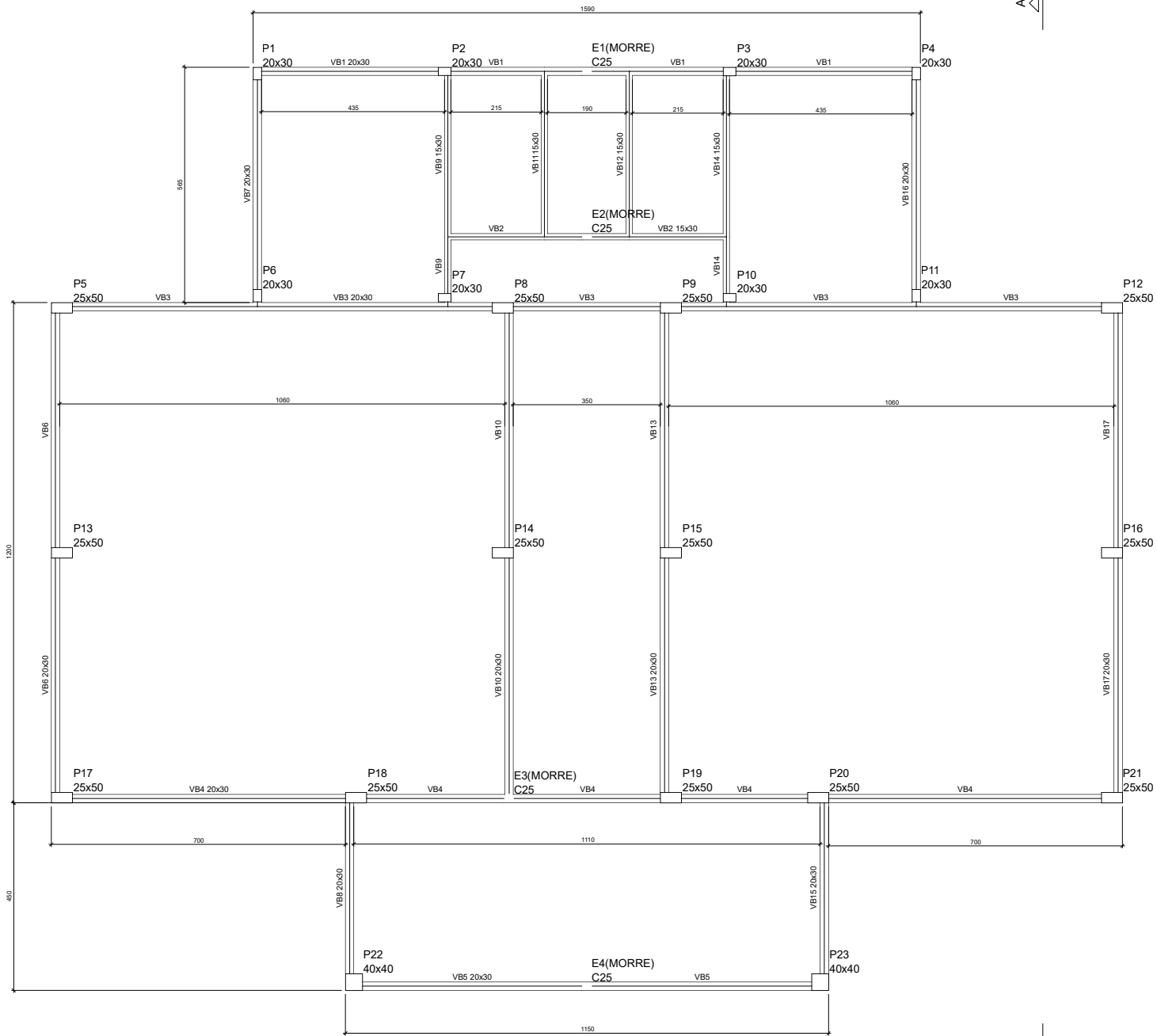
Forma do pavimento Baldrame (Nível 0) escala 1:50
